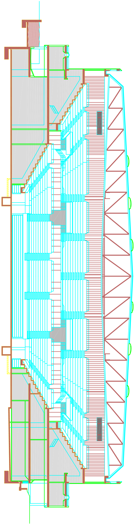
SECCION TRANSVERSAL
